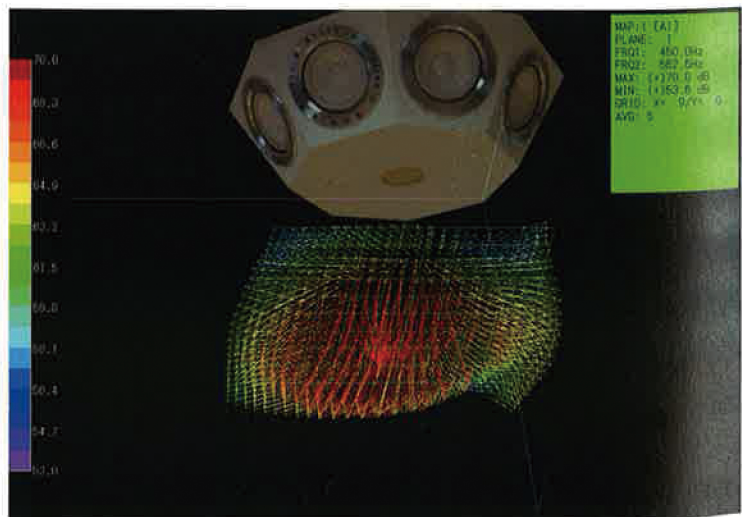
《NS-8master インテンシティ測定結果》
