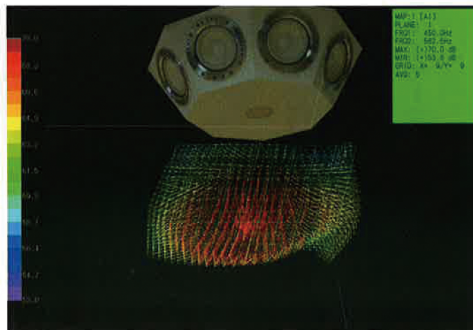
《NS-8master インテンシティ測定結果》
